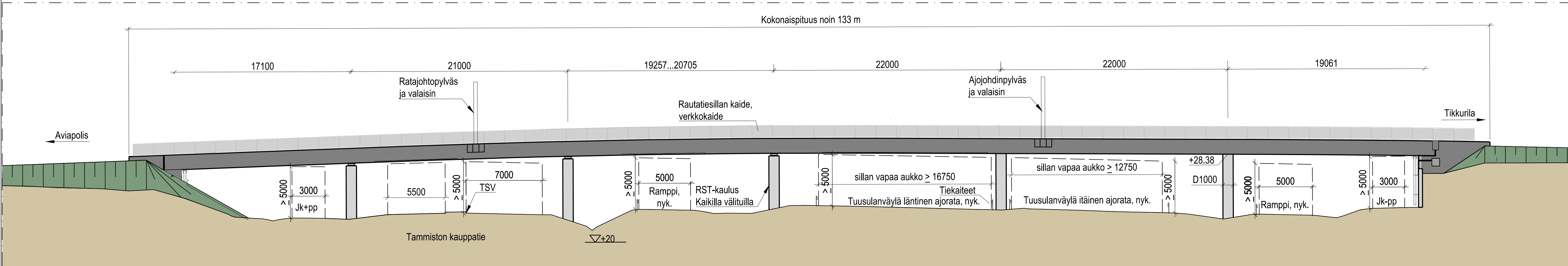
SIVUKUVA A - A 1:200
