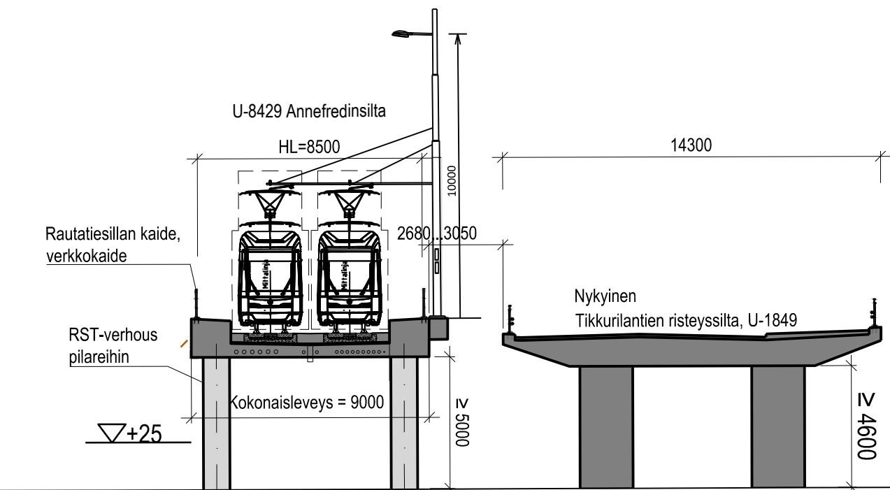
LEIKKAUS B-B 1:200
