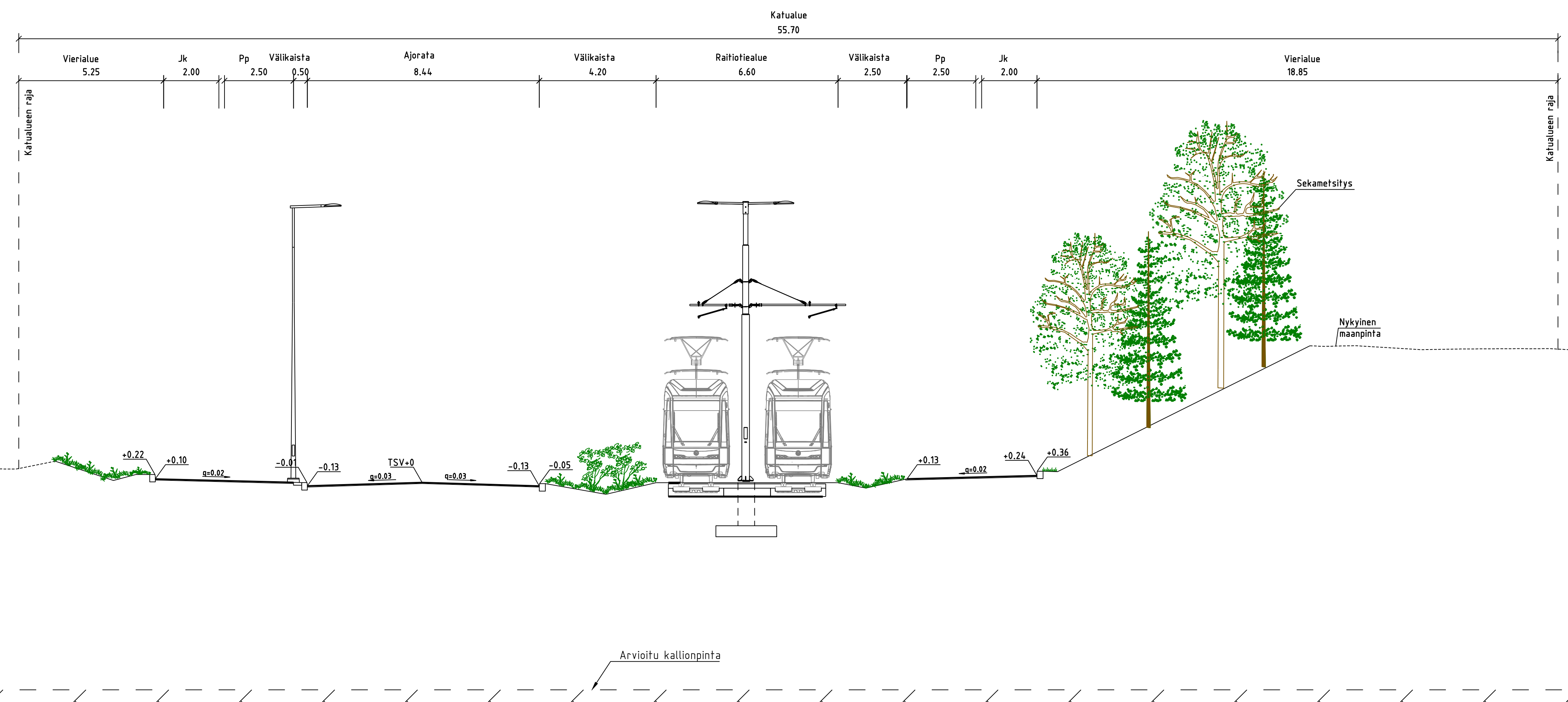
Fazerintie tyypipoikkileikkaus D - D
