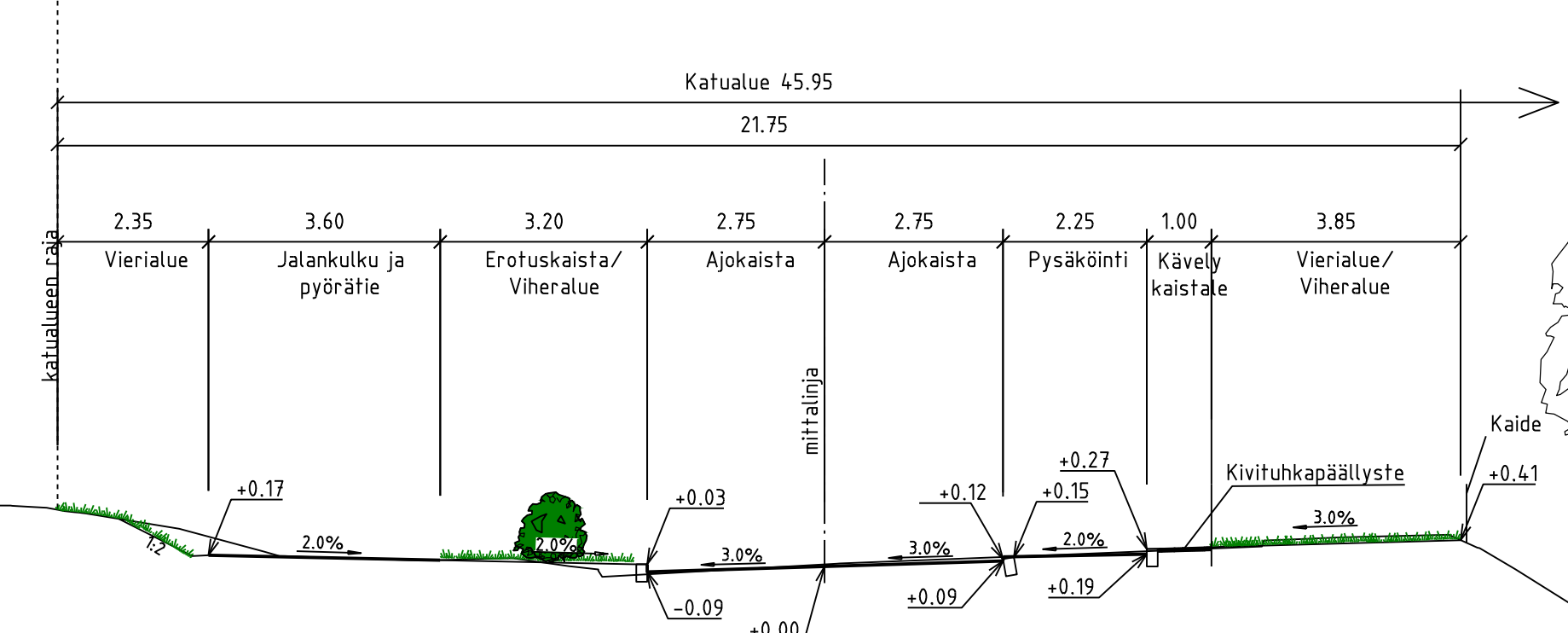
TYYPPIPOIKKILEIKKAUS B-B 1:100
