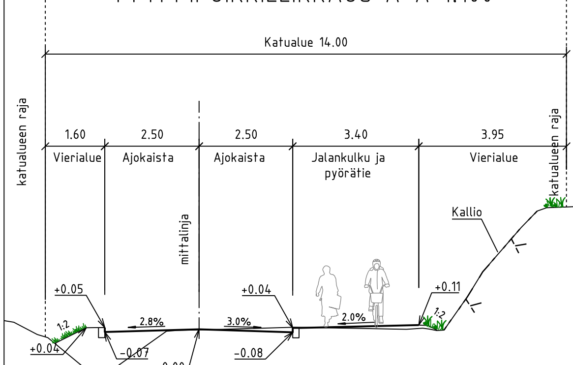
TYYPPIPOIKKILEIKKAUS A-A 1:100
