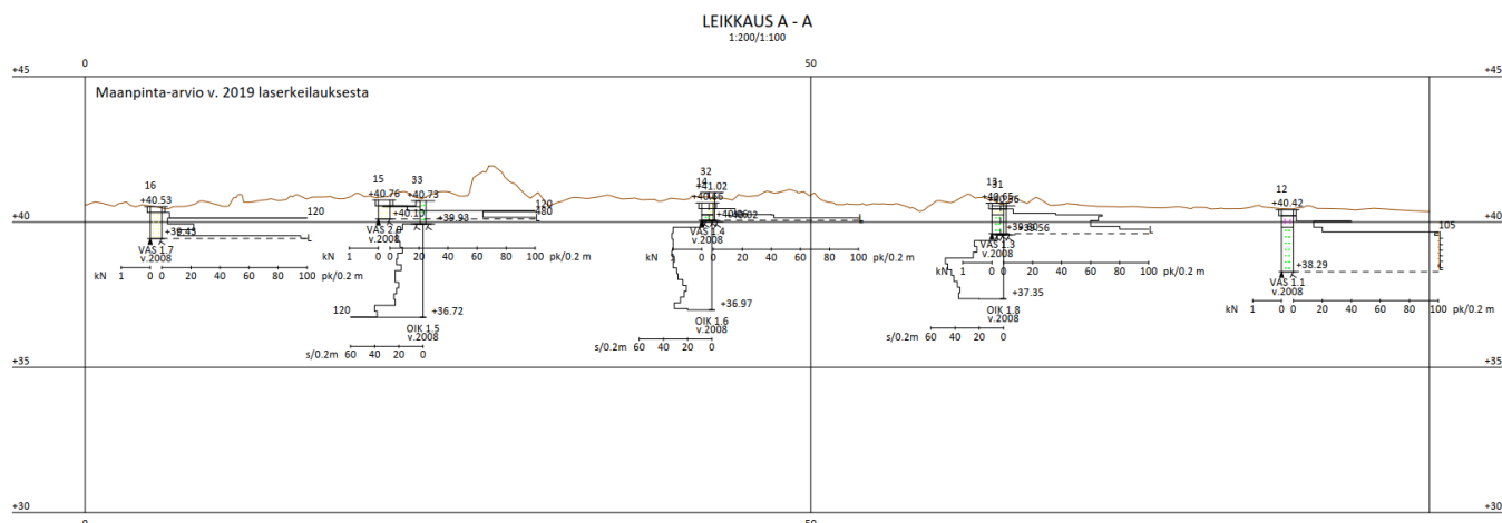
Kuva 2: Leikkaus A-A (ei mittakaavassa!)
