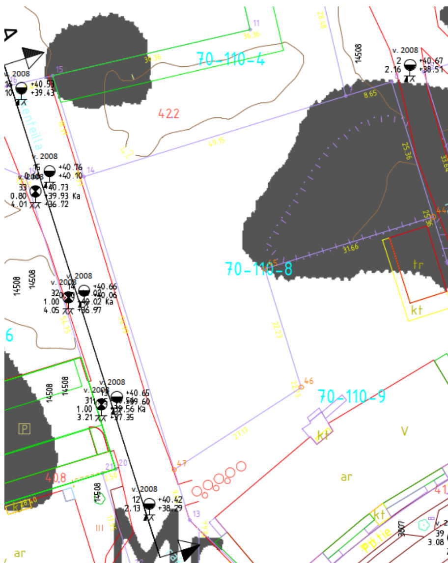
Kuva 1: Maalaji- ja pohjatutkimuskartta (ei mittakaavassa!)
