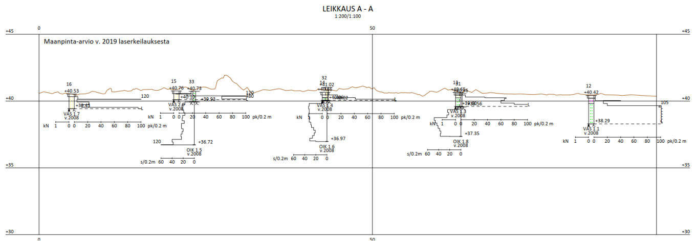
Kuva 2: Leikkaus A-A (ei mittakaavassa!)
