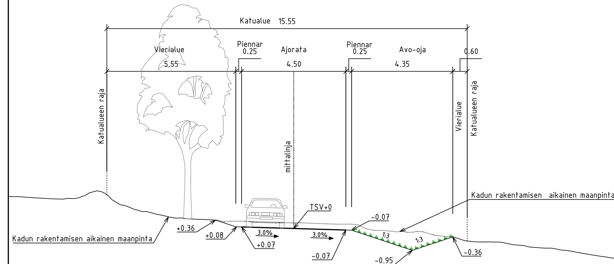
TYYPPIPOIKKILEIKKAUS B-B
