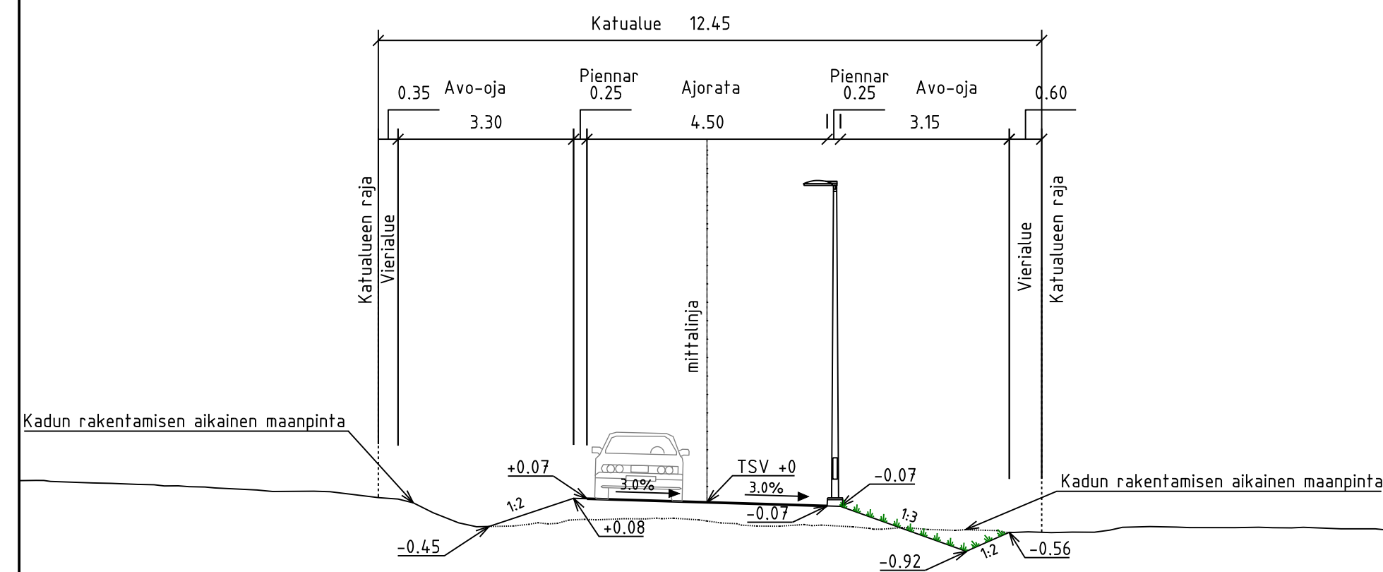
TYYPPIPOIKKILEIKKAUS B-B
