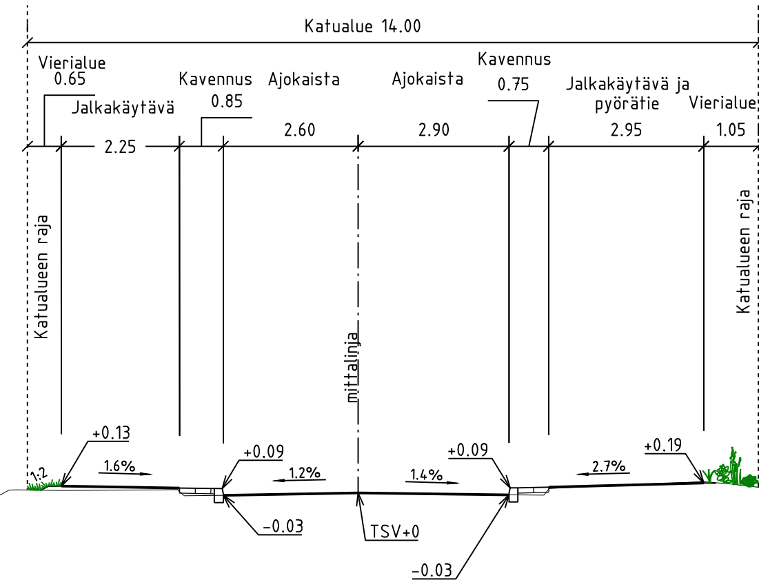
TYYPPIPOIKKILEIKKAUS A-A
