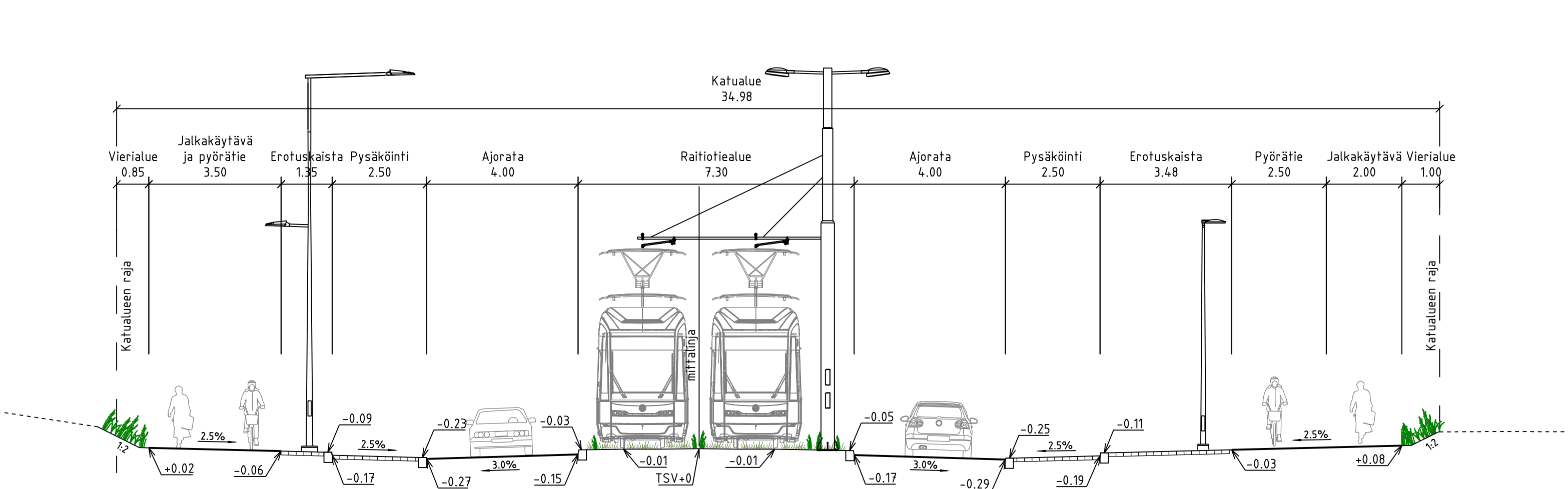
TYYPPIPOIKKILEIKKAUS B-B
