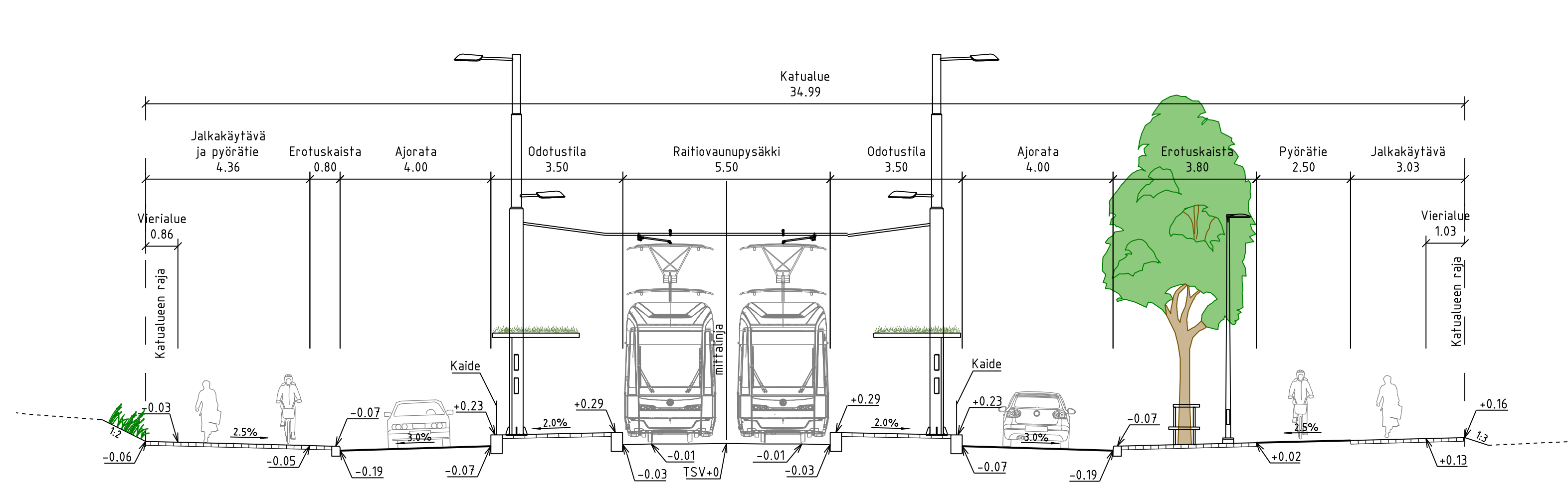
TYYPPIPOIKKILEIKKAUS C-C
