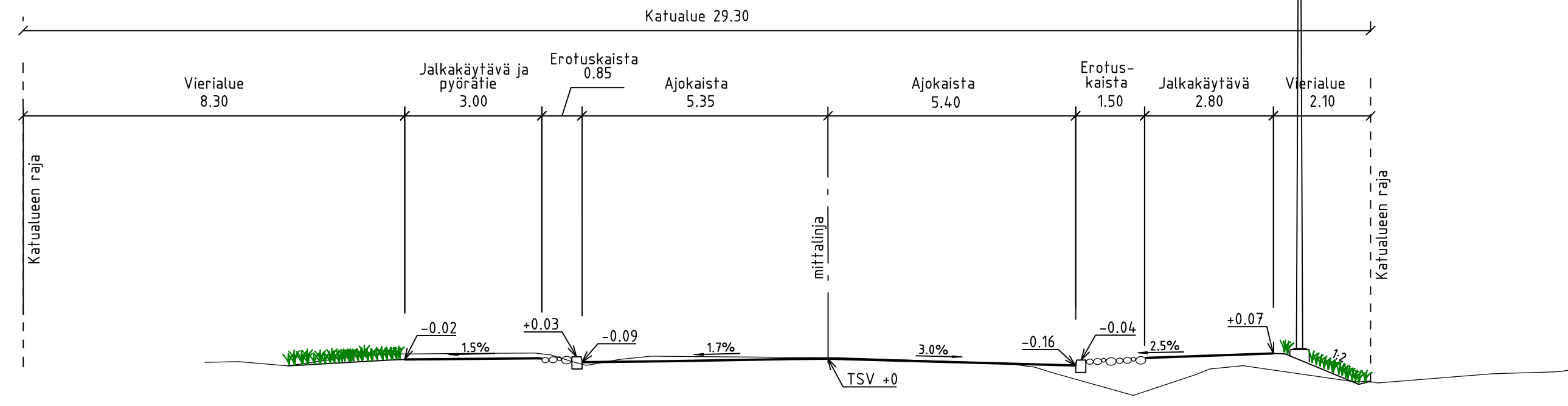
TYYPPIPOIKKILEIKKAUS B-B 1:100
