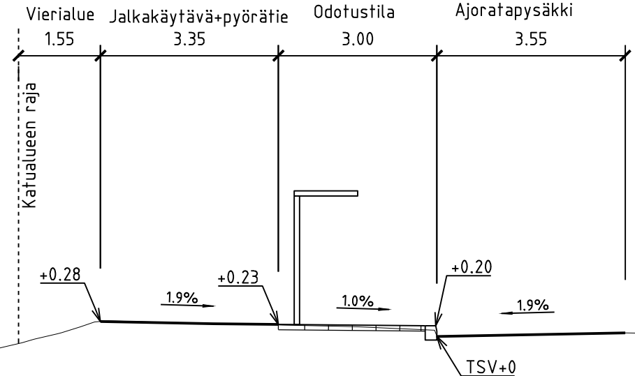
TYYPPIPOIKKILEIKKAUS A-A 1:100
