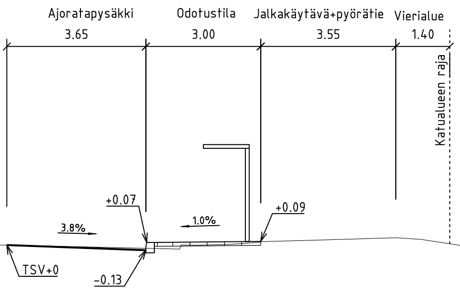
TYYPPIPOIKKILEIKKAUS B-B 1:100
