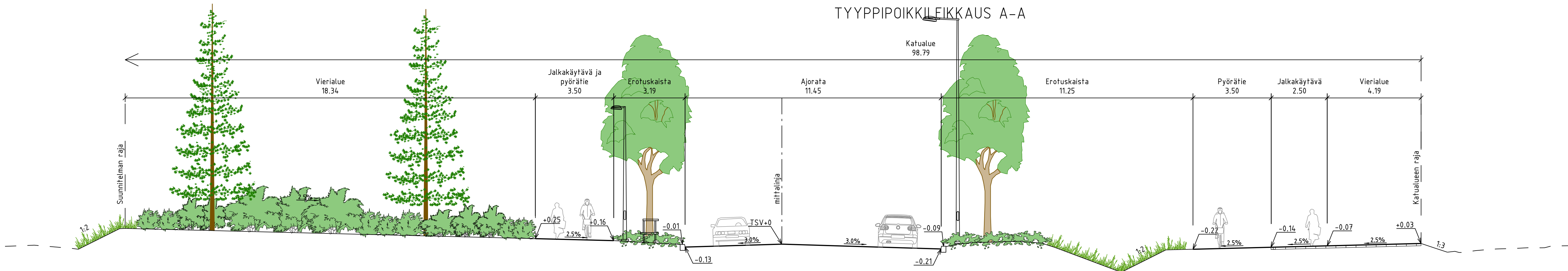
TYYPPIPOIKKILEIKKAUS A-A
