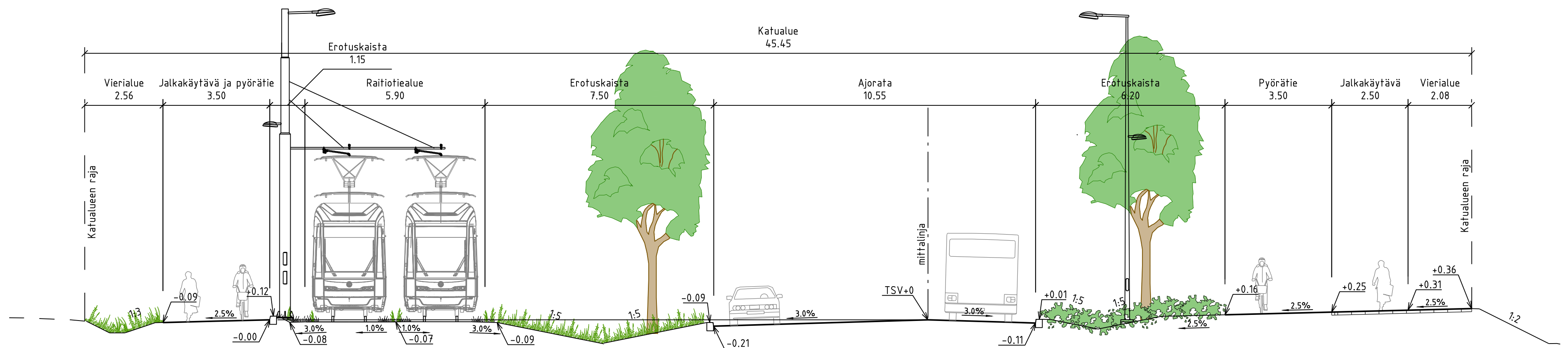
TYYPPIPOIKKILEIKKAUS B-B
