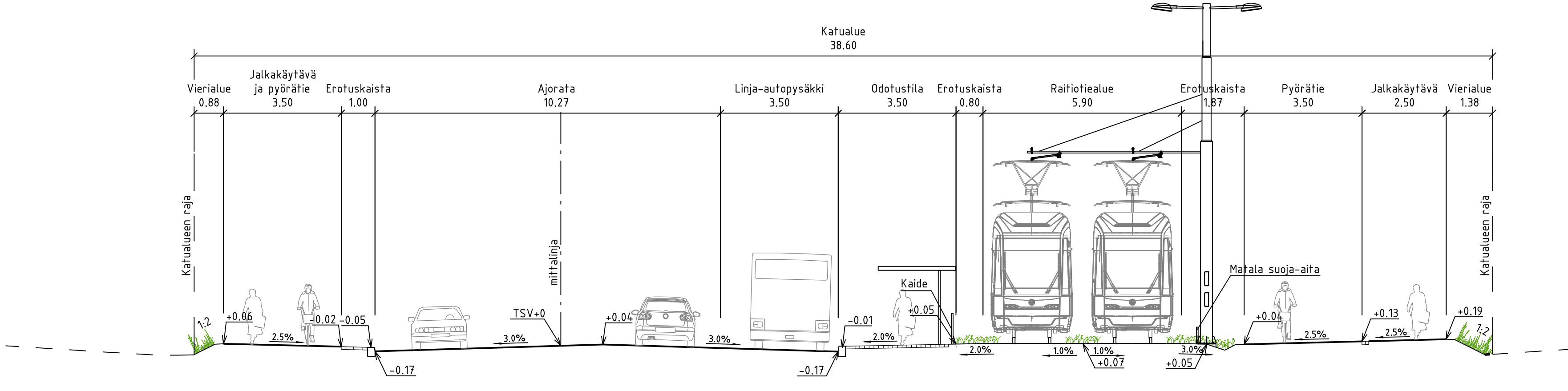
TYYPPIPOIKKILEIKKAUS F-F
