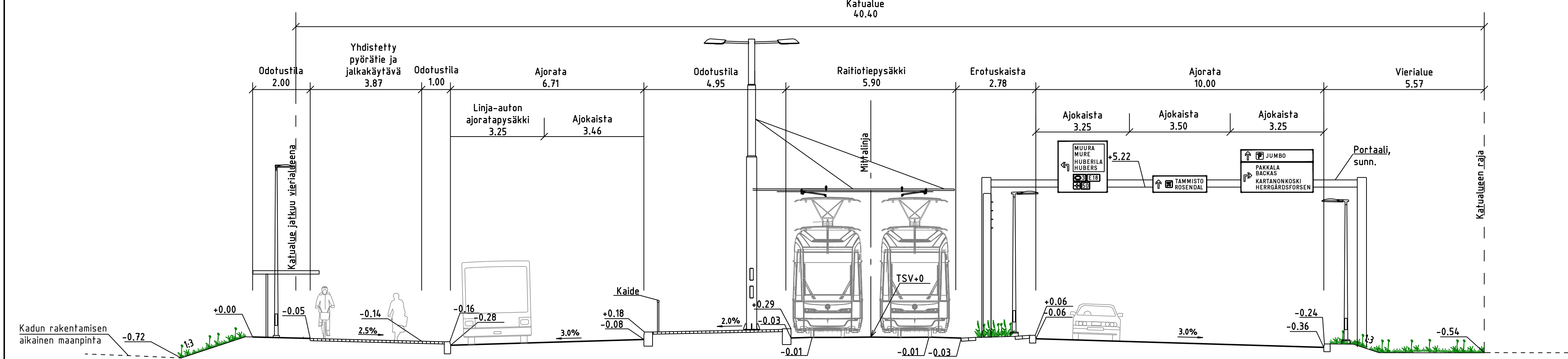
TYYPPIPOIKKILEIKKAUS C-C
