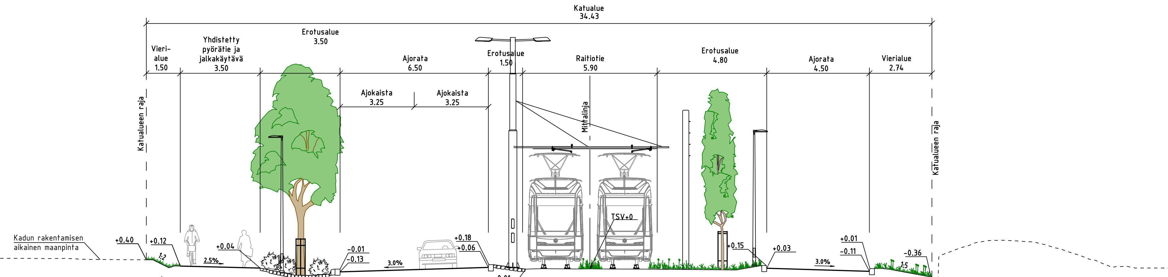
TYYPPIPOIKKILEIKKAUS B-B
