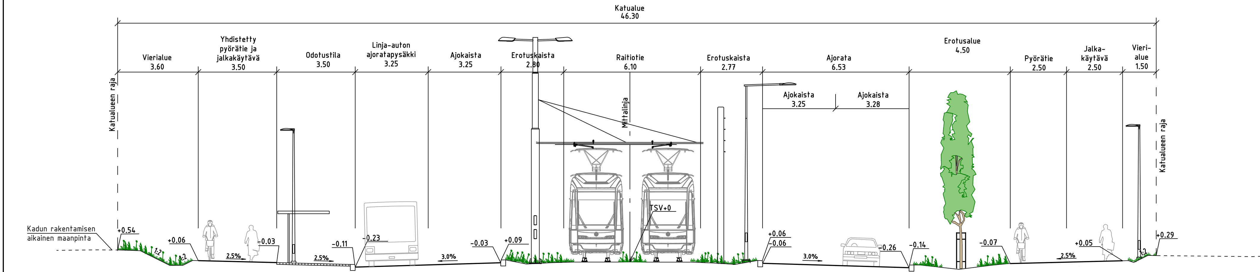
TYYPPIPOIKKILEIKKAUS C-C
